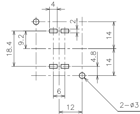
プリント基板用取付穴
